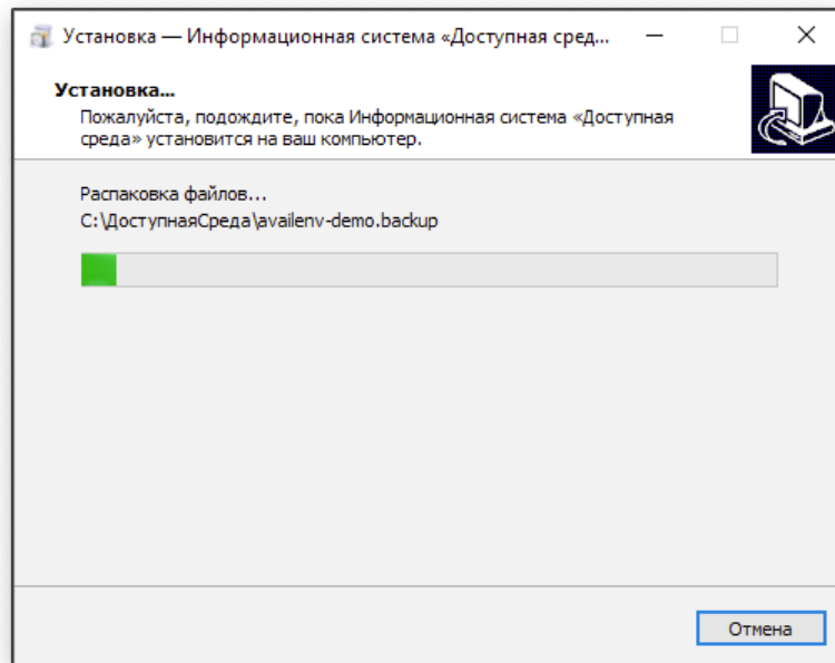
Рис. 4. Процесс установки.
